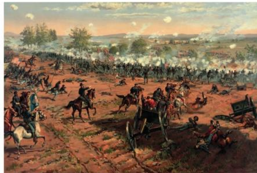
Bitka pri Gettysburgu velja za najbolj krvavo v ameriški državljanski vojni. Na obeh straneh je padlo skoraj 8000 vojakov, ranjenih je bilo več kot 27.000.
